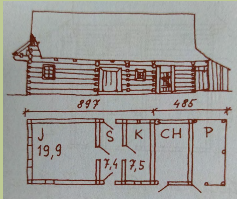
Náčrt chalupy č. 118/ čp. 123
