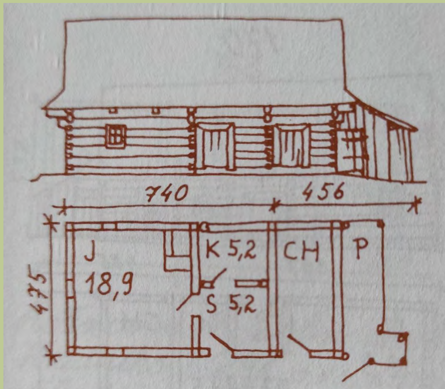
Náčrt chalupy č. 111/čp. 121
